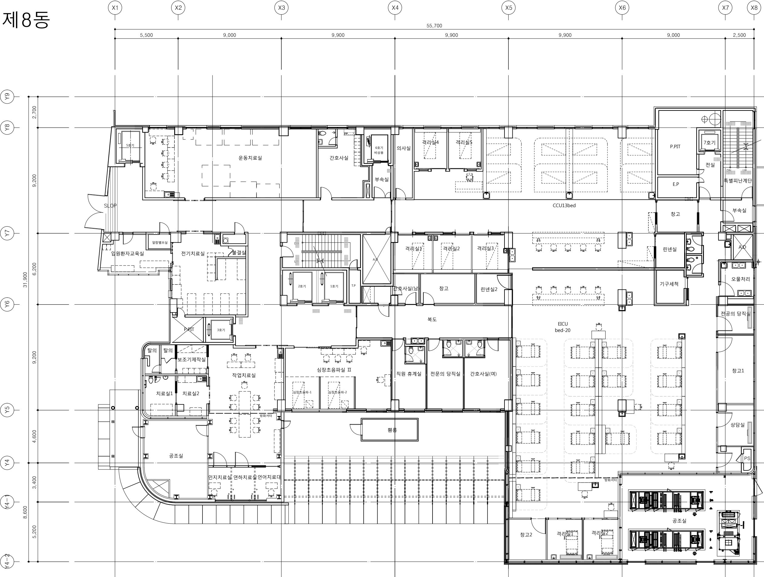
2층 평면도 축척 : 1/100A1, 1/200A3 면적=1,719.73m2
